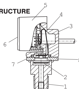
内部構造図
