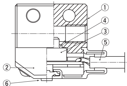
内部構造図 INTERNAL STRUCTURE (2-M5 メネジ 2-M5 female screw)
