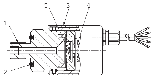
内部構造図 INTERNAL STRUCTURE (G 1/8)
