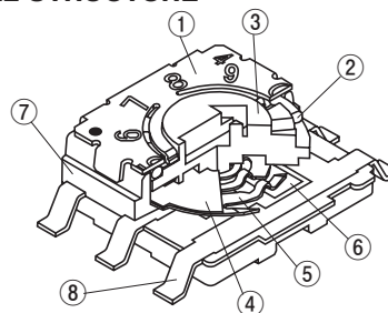
内部構造図 INTERNAL STRUCTURE
